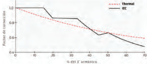
Figura 3.3.3.6. a. Factor de Corrección en función de la proporción de armónicos. Fuente: Adoptada de la norma IEC 60364-5-52.
