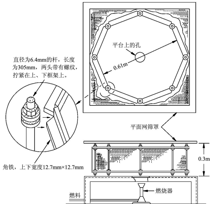
图 B.2 燃烧试验工装
