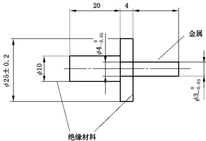
把手的尺寸（ \phi 10 和20）不是关键尺寸。 注：本试验针尺寸为GB/T 16842-2016的图9试验试具13中给出的尺寸，在某些情况下尺寸公差是不同的。
